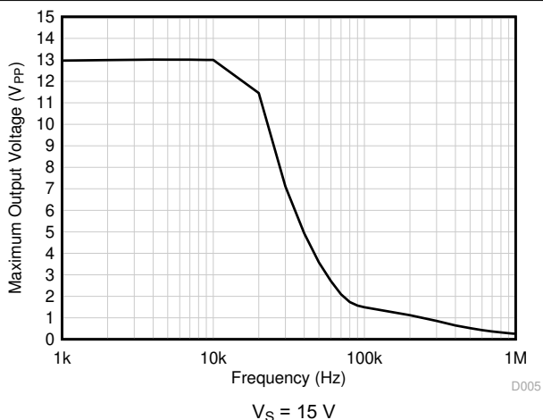
图 5-36. 最大输出电压与频率间的关系
