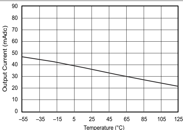
图 5-48. 拉电流限制
