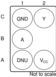
图 4-7. YZP 封装 5 引脚 DSBGA 底视图
