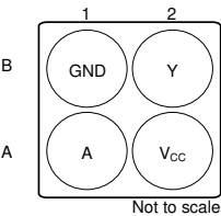
图 4-8. YZV 封装 4 引脚 DSBGA 底视图
